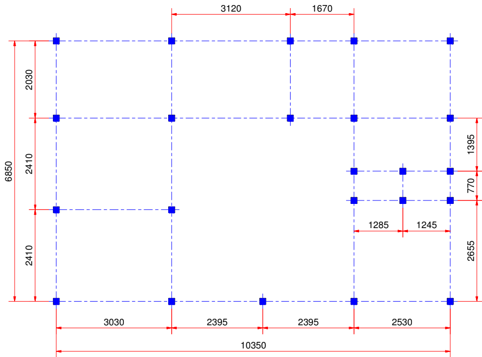
План фундамента (foundation plan)
