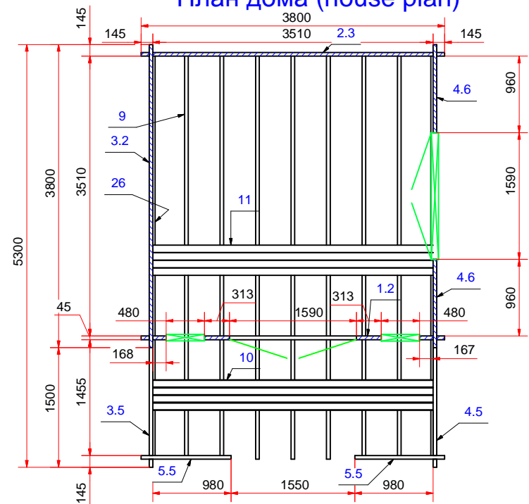
План дома (house plan)
